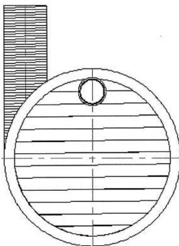
b) montaż kominu stycznie do powierzchni bocznej
