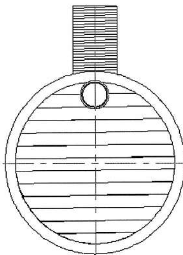
a) montaż kominu w osi zbiornika
