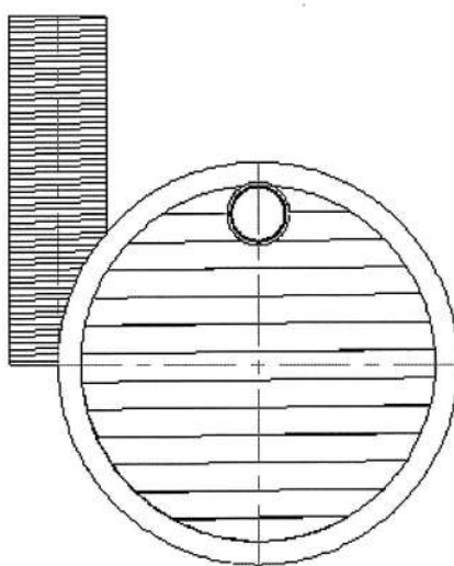
c) montaż kominu ze wsparciem wystającym poza obrys zbiornika
